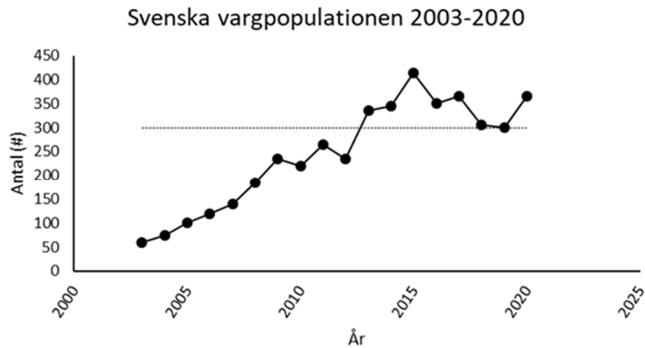
Figur 1. Utveckling av den svenska vargstammen 2003-2020 12 .
