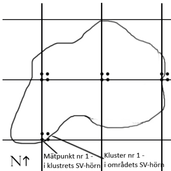
Figur 4. Schematisk bild som visar kluster av mätpunkter som placerats ut över ett rikkärrområde. Området är 7,8 ha stort och det är 154,91 m mellan maskorna i rutnätet. I alla maskor vars SV-hörn hamnar inom området (4 st på bilden) placeras ett kluster med mätpunkter. Alla mätpunkter som faller inom rikkärrets avgränsning (13 st) ska undersökas. Några av mätpunkterna kan komma att strykas i fält.
