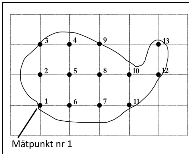
Figur 2. Schematisk bild över en grid av mätpunkter i ett rikkärr. Det är lika långt mellan mätpunkterna (svarta punkterna) i nord-sydlig riktning som i öst-västlig. Mätpunkt nr 1 är den som ligger längst västerut och längst söderut i rikkärret. Antalet mätpunkter i figuren är 13 men några mätpunkter kan komma att strykas i fält. Vid semipermanenta provytor ökas antalet mätpunkter med 30 %.
