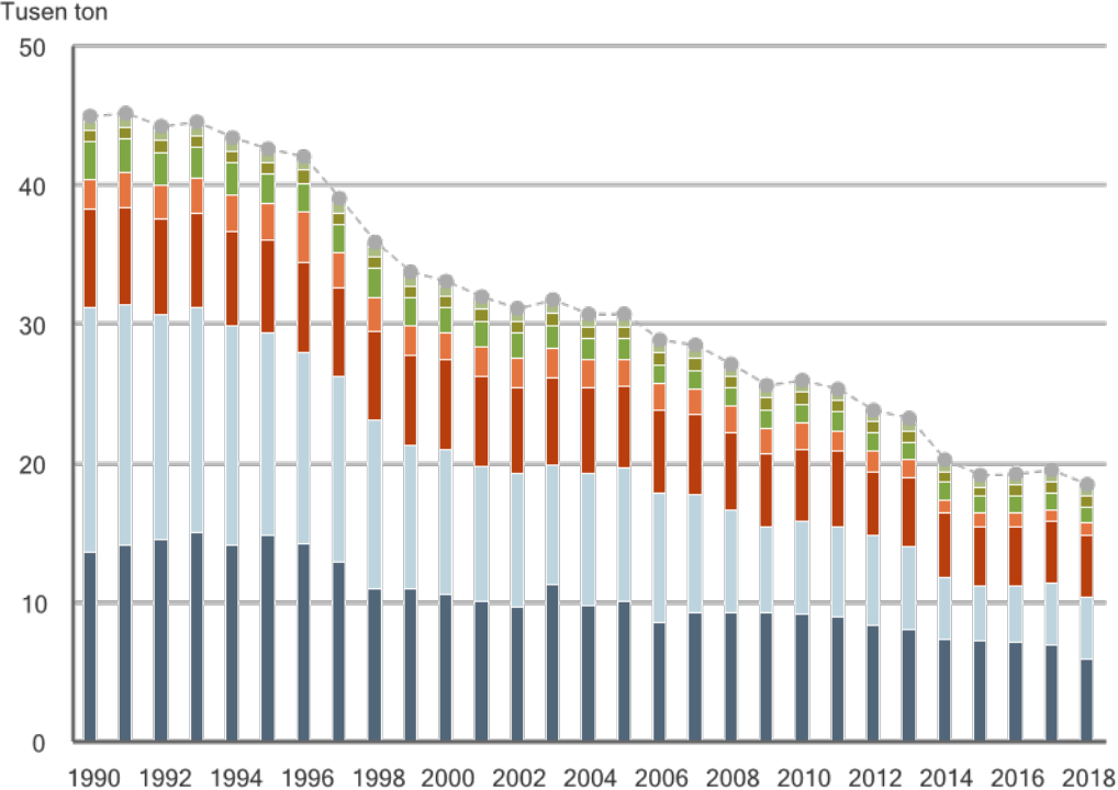
Utsläpp av små partiklar (PM 2,5 ) till luft 1990-2018
