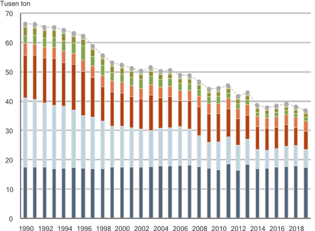
Utsläpp av grova partiklar (PM10) till luft 1990-2019
