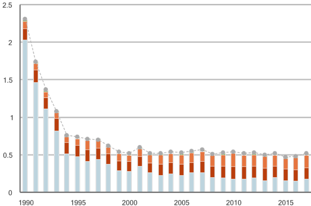
Utsläpp av kadmium till luft 1990-2017
