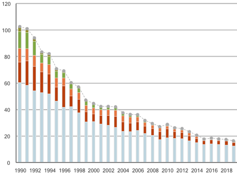
Utsläpp av svaveldioxidutsläpp till luft 1990-2019
