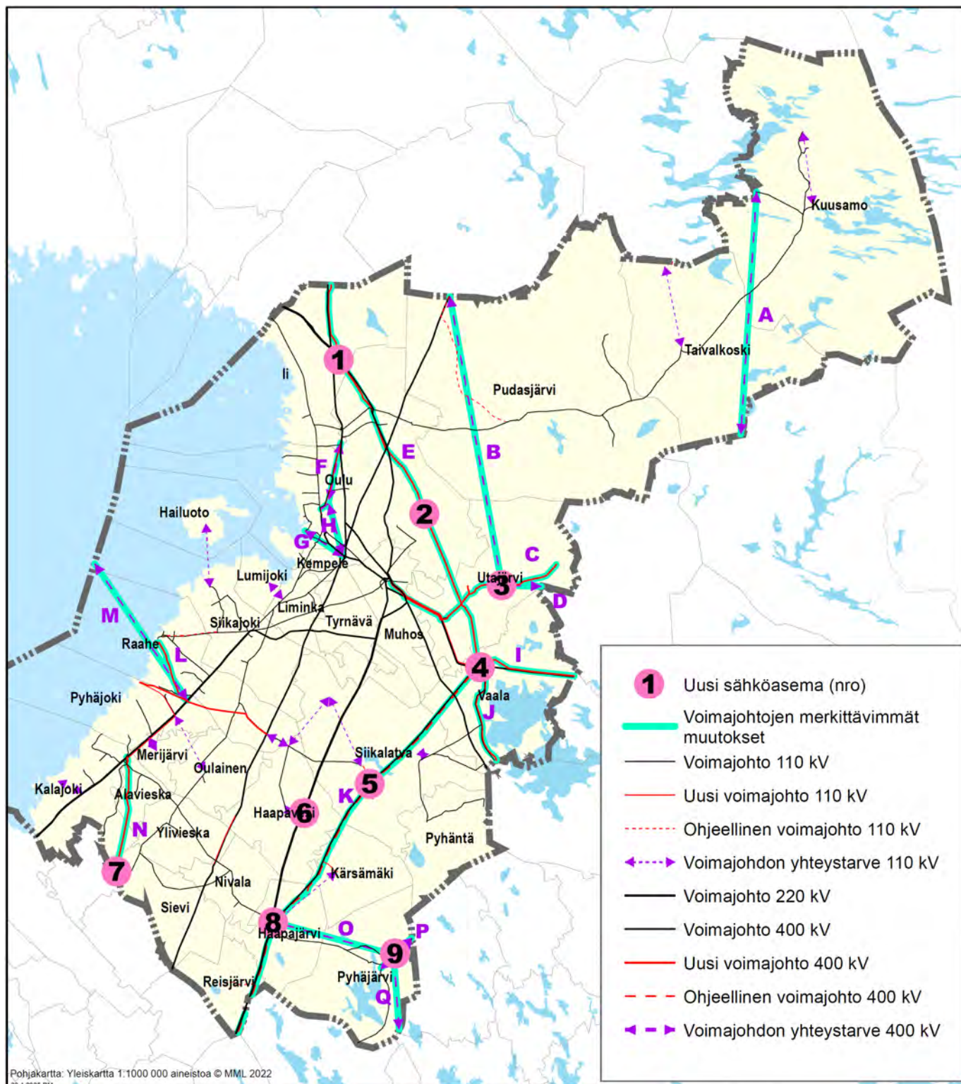
Bild 27. Etapplandskapsplanens elöverföringslösningar och mest betydande förändringar i förhållande till gällande landskapsplaner. Med turkos anges de största kända förändringarna. Elstationer: 1=Herva, 2=Vuotto, 3=Pontema, 4=Nuojuankangas, 5=Siikalatva, 6=Pihtineva, 7=Kukonkylä, 8=Pysäysperä, 9=Murtoperä. Kraftlednigarnas koder anges i föregående tabell.
