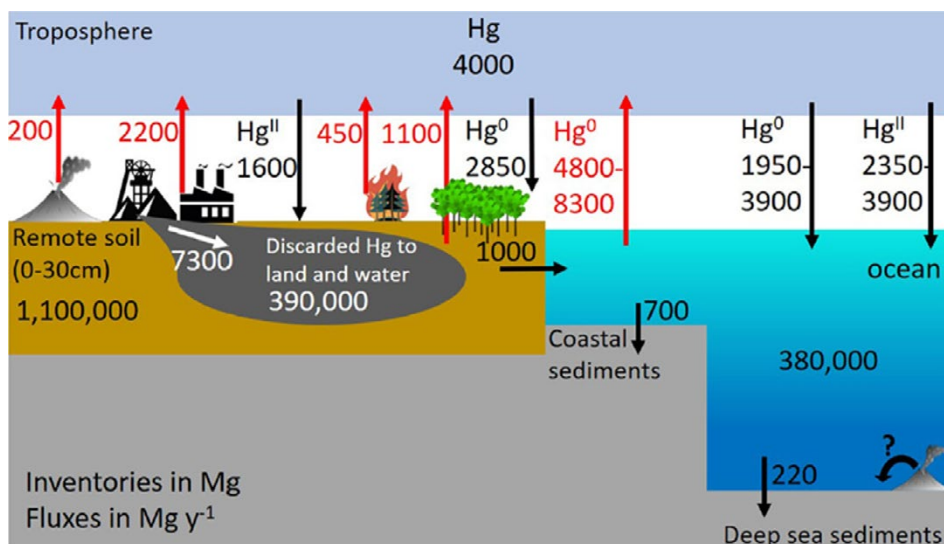
Figur 1. Nutida global budget för kvikksilvrets kretslopp vid jordens yta i form av ackumulerade pooler (Inventories) uttryckt i megagram (Mg, 1 Mg = 1 ton) och flöden (Fluxes) uttryckt i megagram per år (Mg y -1 ). Emissioner till atmosfären visas med röda pilar och övriga flöden med svarta pilar. Reproducerad från Sonke et al. (Sonke et al., 2023) i enlighet med upphovsrättslicens CC BY 4.0.
