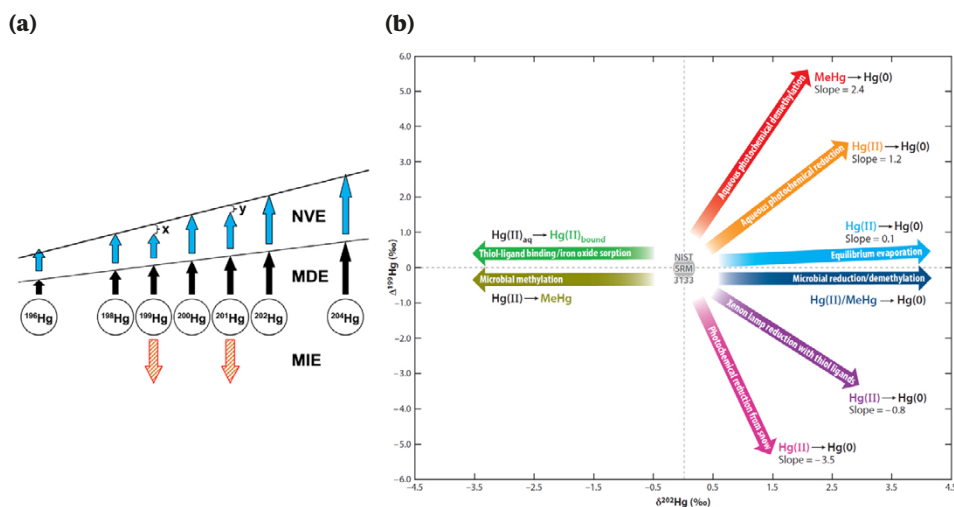
Figur 7. (a) Schematisk illustration av fraktioneringsmekanismer i kvicksilvrets isotopsystem. Pilarna anger på ett kvalitativt sätt påverkan av masskillnadseffekter (mass-dependent effect, MDE), kärnvolyms effekter (nuclear volume effect, NVE) samt magnetiska isotop-effekter (magnetic isotope effect, MIE) på de sju stabila kvicksilverisotoperna. Reproducerad från Wiederhold (Wiederhold, 2015) i enlighet med upphovsrättslicens CC BY 4.0. (b) Översikt över experimentellt observerade generella mönster i isotopfraktionering för kvicksilver. Pilarna visar riktningen för isotopfraktioneringen hos reaktanterna eller produkterna enligt färgkodningen. Reproducerad från Blum et al. (Blum et al., 2014) i enlighet med upphovsrättslicens CC BY 4.0.
