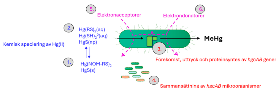
Figur 3. Illustrering av kända nyckelfaktorer som styr hgc -driven mikrobiell metylering av oorganiskt tvåvärt kvikksilver (Hg(II)) till metylkvikksilver (MeHg). Kemisk speciering av Hg(II) i (1.) fast fas respektive (2.) löst i vatten; (3.) Förekomst (abundans), uttryck (transkript) och proteinsyntes (translation) av hgcAB gener; (4.) Taxonomisk sammansättning av mikroorganismer som bär på hgcAB gener; (5.) Tillgång på anaeroba mikrobiella elektronacceptorer (trevärt järn, sulfat, koldioxid); (6.) Tillgång på anaeroba mikrobiella elektronondonatorer (organiska kolföreningar).
