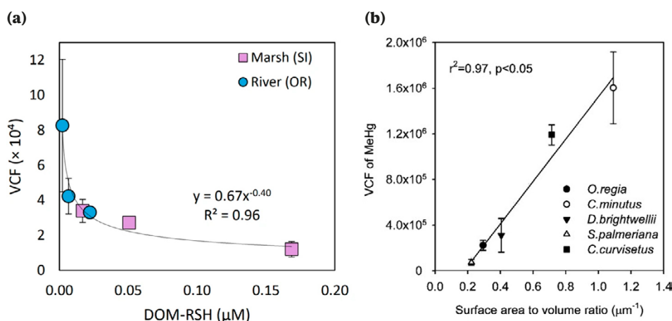
Figur 6. (a) Anrikning av metylkvicksilver i den marina diatomen Thalassiosira pseudonana , uttryckt som volymkoncentrationsfaktor (VCF), som funktion av koncentrationen tiolföreningar i löst organiskt material (DOM-RSH) för två olika akvatiska miljöer (marsh, river). Reproducerad från Seelen et al. (Seelen et al., 2023) i enlighet med upphovsrättslicens CC BY 4.0. (b) Anrikning av metylkvicksilver i fem olika växtplankton organismer, uttryckt som volymkoncentrationsfaktor (VCF), som funktion av planktoncellernas ytarea-till-volym-förhållande. Reproducerad från Kim et al. (Kim et al., 2014) i enlighet med upphovsrättslicens CC BY 4.0.
