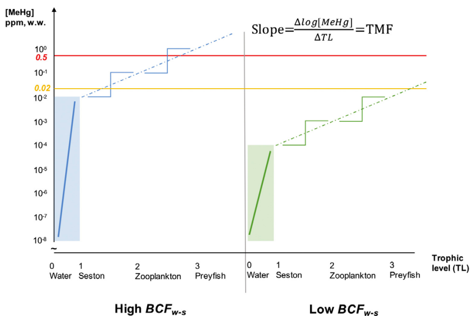
Figur 5. Konceptuell illustration av anrikning av metylkvicksilver från vatten till den lägsta trofinivån (seston) i den pelagiska näringsväven, uttryckt som biokoncentrationsfaktor (BCF), samt vidare anrikning med ökande trofinivå i näringsväven, uttryckt som trofisk anrikningsfaktor (trophic magnification factor, TMF). Den horisontella orangefärgade linjen visar EUs gränsvärde på 0.02 µg Hg g -1 våtvikt i biota och den horisontella rödfärgade linjen visar WHO:s gränsvärde på 0.5 µg Hg g -1 våtvikt i fisk. Reproducerad från Wu et al. (Wu et al., 2019) i enlighet med upphovsrättslicens CC BY 4.0.
