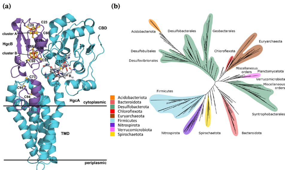
Figur 4. (a) Modellstruktur för enzymkomplexet HgcAB. HgcA visas i blågrått och HgcB i lila. Molekylstrukturerna för det aktiva metyleringscentrumet ( B_{12} ) i HgcA och järn-svavelklustren (cluster A, cluster B) i HgcB illustreras mer detaljerat. Reproducerad från Cooper et al. (Cooper et al., 2020) i enlighet med upphovsrättslicens CC BY 4.0. (b) förenklat fylogenetiskt träd för hgcA gensekvenser detekterade i mikroorganismer från miljöprover registrerade i Hg-MATE databasen. Reproducerad från Capo et al (Capo et al., 2023) i enlighet med upphovsrättslicens CC BY 4.0.
