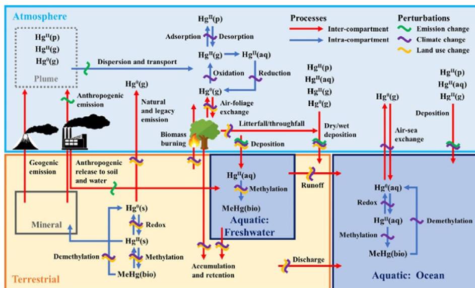
Figur 2. Nyckelprocesser av betydelse för kvikksilvrets globala kretslopp, inklusive flöden mellan centrala miljömedier. Figuren illustrerar även vilka processer och flöden som kan påverkas av förändringar i kvikksilverutsläpp (Emission change), klimat (Climate change) och markanvändning (Land use change). Reproducerad från Obrist et al. (Obrist et al., 2018) i enlighet med upphovsrättslicens CC BY 4.0.
