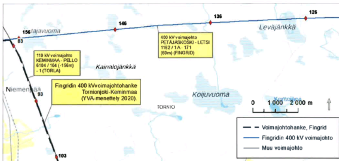
Kuva 1. Voimajohtodot alueella.
