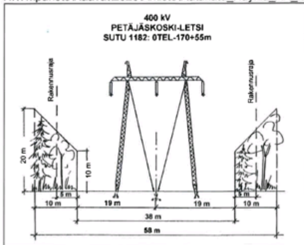
Kuva 2. Fingridin 400 kV voimajohdon Petäjäskoski - Letsi poikkileikkaus.
