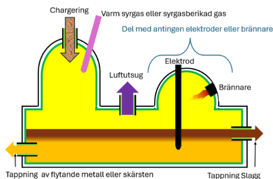
Figur 37: Principskiss av flashugn i genomskärning
