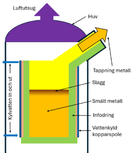
Figur 31: Induktionsugn med spole runt degeln i genomskärning.
