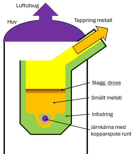
Figur 30: Induktionsugn av rännungstyp i genomskärning.
