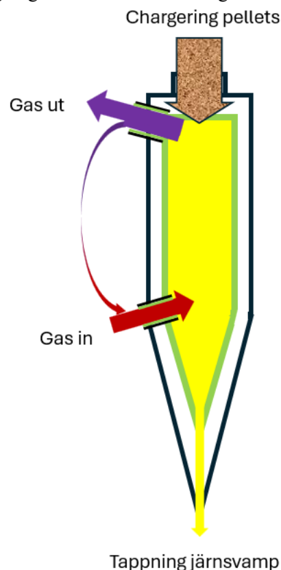
Figur 22; Schaktugn för järnframställning i genomsnitt.
