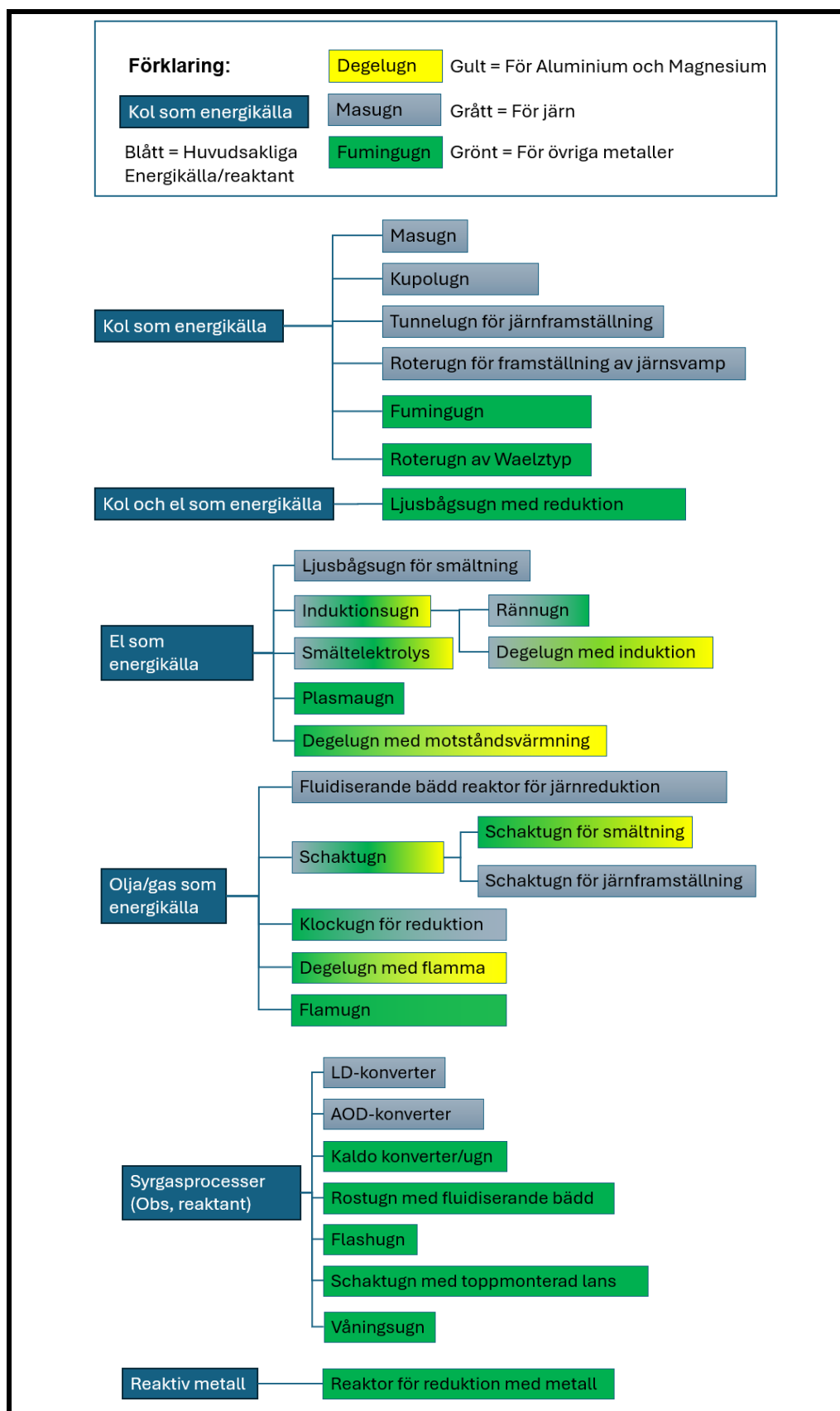
Figur 16: Ugnsindelning efter reaktant/energikälla och vilka metaller de används till.
