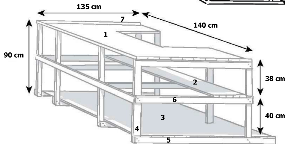
Figur 6. Skjutstol med skjutstöd. Mått och konstruktion är att se som exempel.
