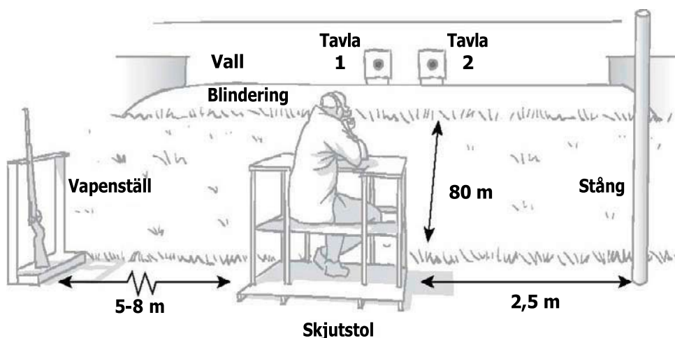
Figur 5. Exempel. Provplats för säker vapenhantering och precisionsskjutning. Provplats för säker vapenhantering och precisionsskjutning. Måtten mellan vapenställ, skjutstol och stång är ungefärliga.
