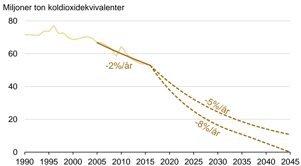
Figur 1: Minskningstakt för 2005–2016 samt genomsnittliga minskningstakter för att nå netto-nollmålet till 2045. Källa: Naturvårdsverket, 2017f
