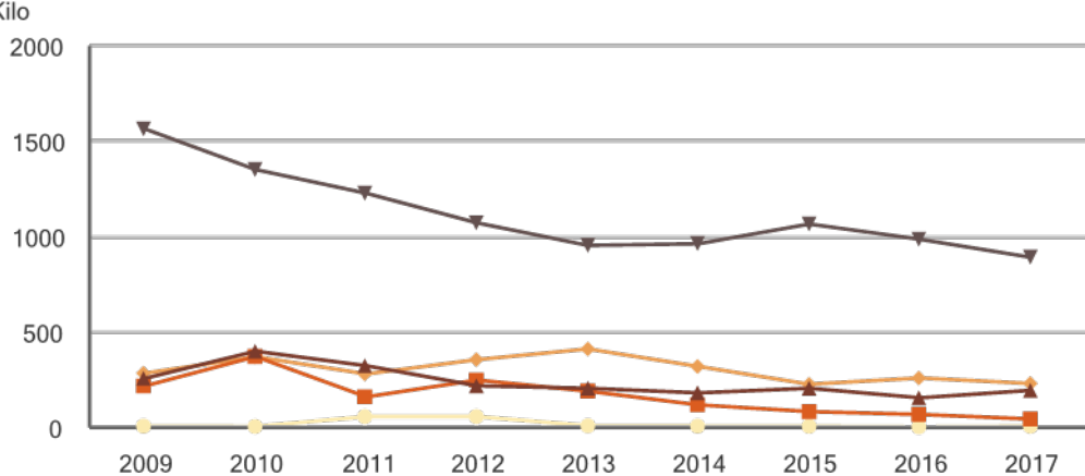
Utsläpp av bly från industrianläggningar till vatten 2009-2017
