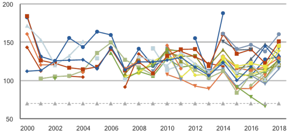
Maximala 8-timmarsmedelvärden av ozon i gaturum och urban bakgrund 2000-2018
