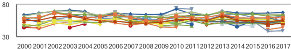
Årsmedelhalter av ozon i urban och regional bakgrund 2000-2017
