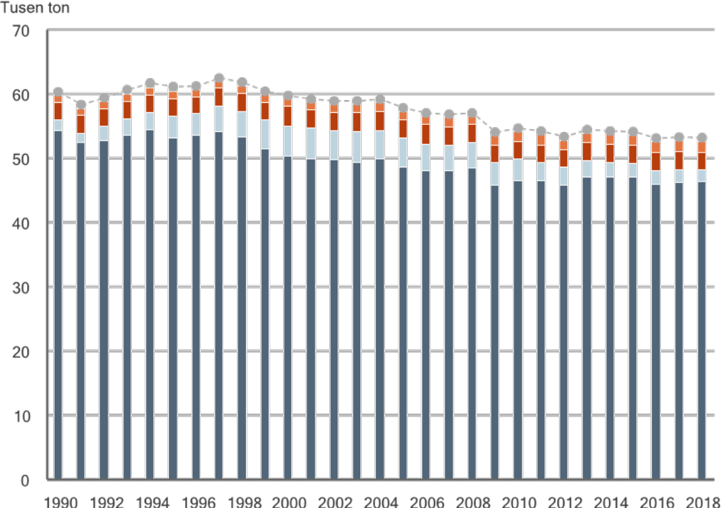
Utsläpp av ammoniak till luft 1990-2018
