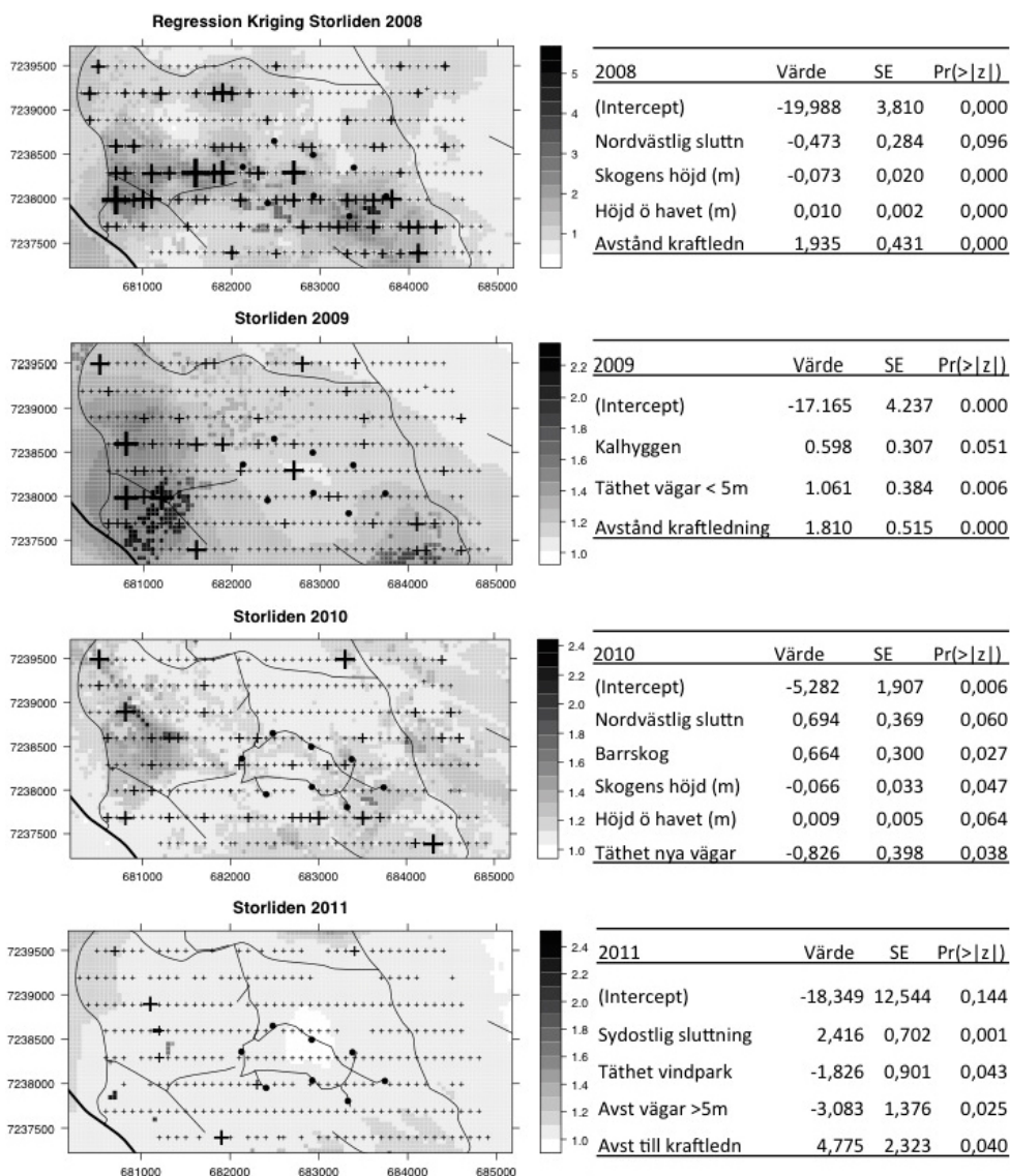
Figur 7. Kartor över predikterad utbredning av renspillning i Storliden för 2008-2011, observera att kartan för 2008 baseras på orensade ytor. Värdena i tabellerna är de skattade regressionsvärden från GLM-modellen för respektive år med standardfelet och p-värdet angivet. Kryssen (+) på kartan markerar var inventeringspunkterna ligger och dess storlek är relaterad till antal högar som är hittade på platsen, cirklarna (•) markerar var vindkraftverken är byggda (uppförda under 2011), och linjerna markerar var vägarna går i området, de nya vägarna är endast utritade efter det att de började byggas.
