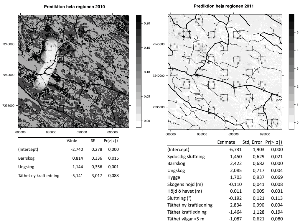
Figur 6. Kartor över predikterad utbredning av renspilling i Jokkmokksliden för år 2010 och 2011 (rensade ytor), de år som parkerna byggdes. Värdena i tabellerna är de skattade regressionsvärden från GLM-modellen för respektive år. Kryssen (+) på kartan markerar var inventeringspunkterna ligger och dess storlek är relaterad till antal högar som är hittade på platsen, cirklarna (●) markerar var vindkraftverken är byggda (uppförda under 2011), och linjerna markerar var vägarna går i området, de nya vägarna är endast utritade efter det att de började byggas.
