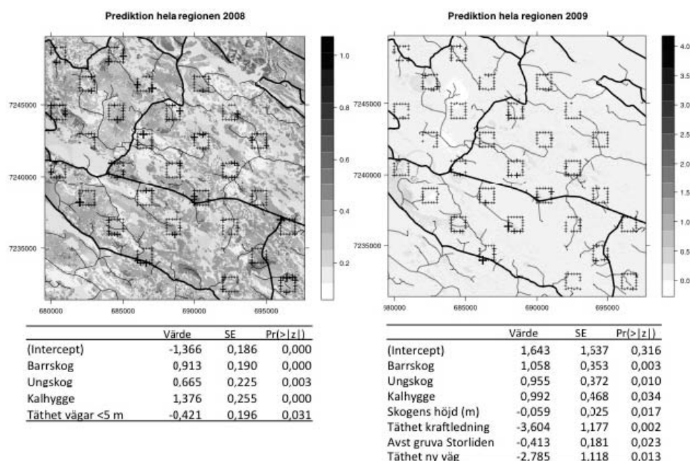
Figur 5. Kartor över predikterad utbredning av renspilling i hela studieområdet för år 2008 (orensade ytor) och 2009 (rensade ytor), före byggnation. Värdena i tabellerna är de skattade regressionsvärden från GLM-modellen för respektive år. Kryssen (+) på kartan markerar var inventeringspunkterna ligger och dess storlek är relaterad till antal högar som är hittade på platsen, cirklarna (●) markerar var vindkraftverken är byggda (uppförda under 2011).
